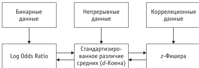
Рис. Конвертация между различными величинами эффектов 1
